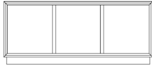
ART. C33/P BASE con 3 ante. cm. l. 163 p. 37 h. 66
