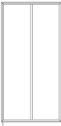
ART. C1/P COL. doppia SX. ART. C2/P COL. doppia DX. cm. l. 110 p. 37 h. 225
