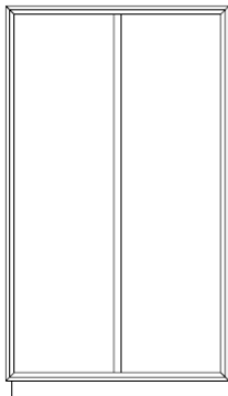
ART. C45/P COL. doppia SX. ART. C46/P COL. doppia DX. cm. l. 110 p. 37 h. 172
