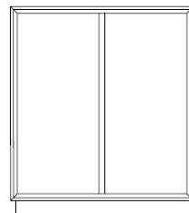
ART. C51/P COL. doppia SX. ART. C52/P COL. doppia DX. cm. l. 110 p. 37 h. 119
